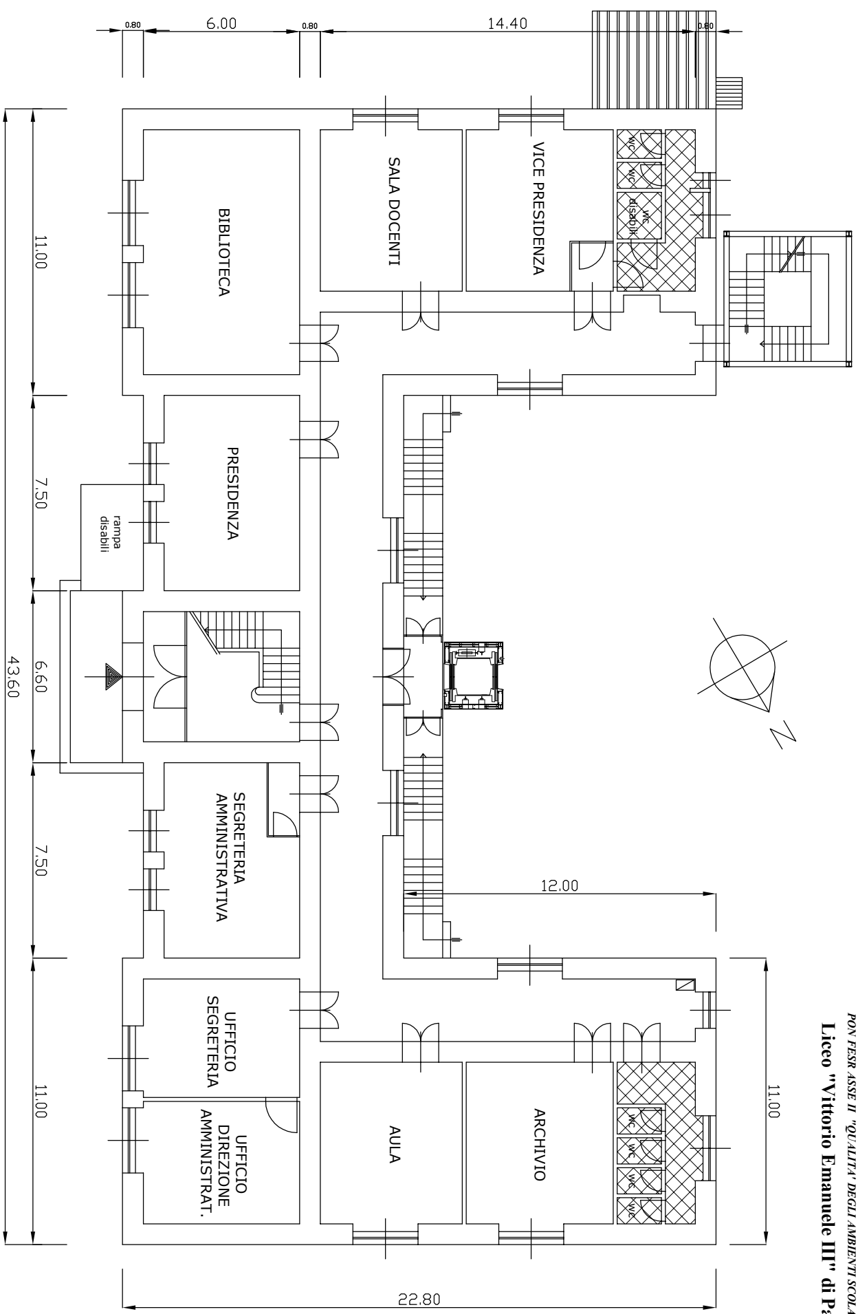
PIANTA PIANO TERRA - rapp. 1:200
